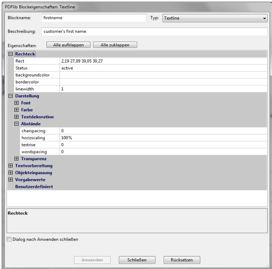
Abb. 13.2 Dialog PDFlib-Blockeigenschaften
